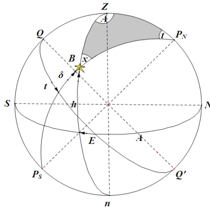
图 4 天体三角形
